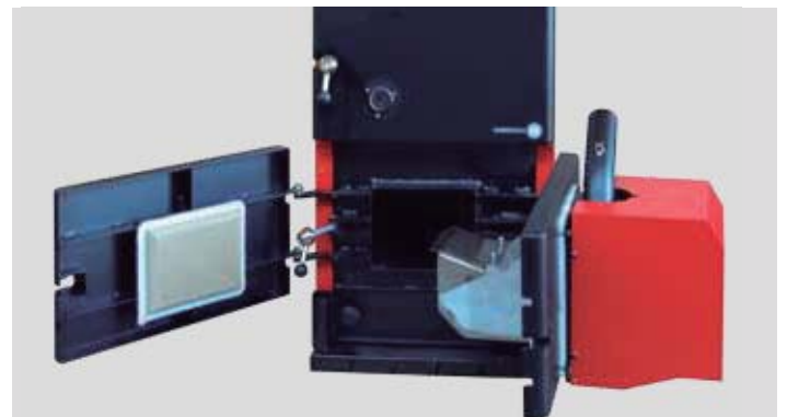
EJEMPLO DE CALDERA CON FUNCIONAMIENTO A PELLET Y A LEÑA CON DOBLE PUERTA.
